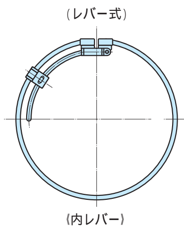
内レバー式バンド
